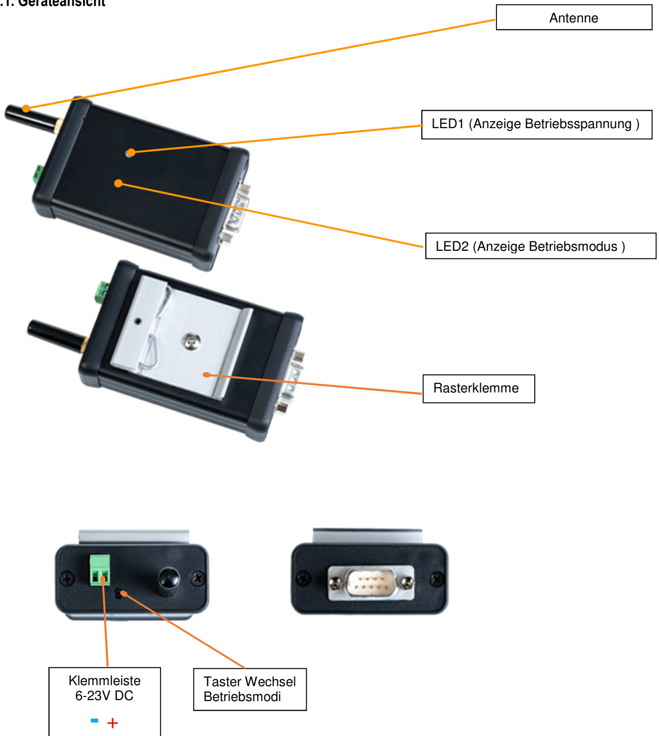
Abbildung 1 Geräteansichten Bluetooth ® RS232 HS Adapter
