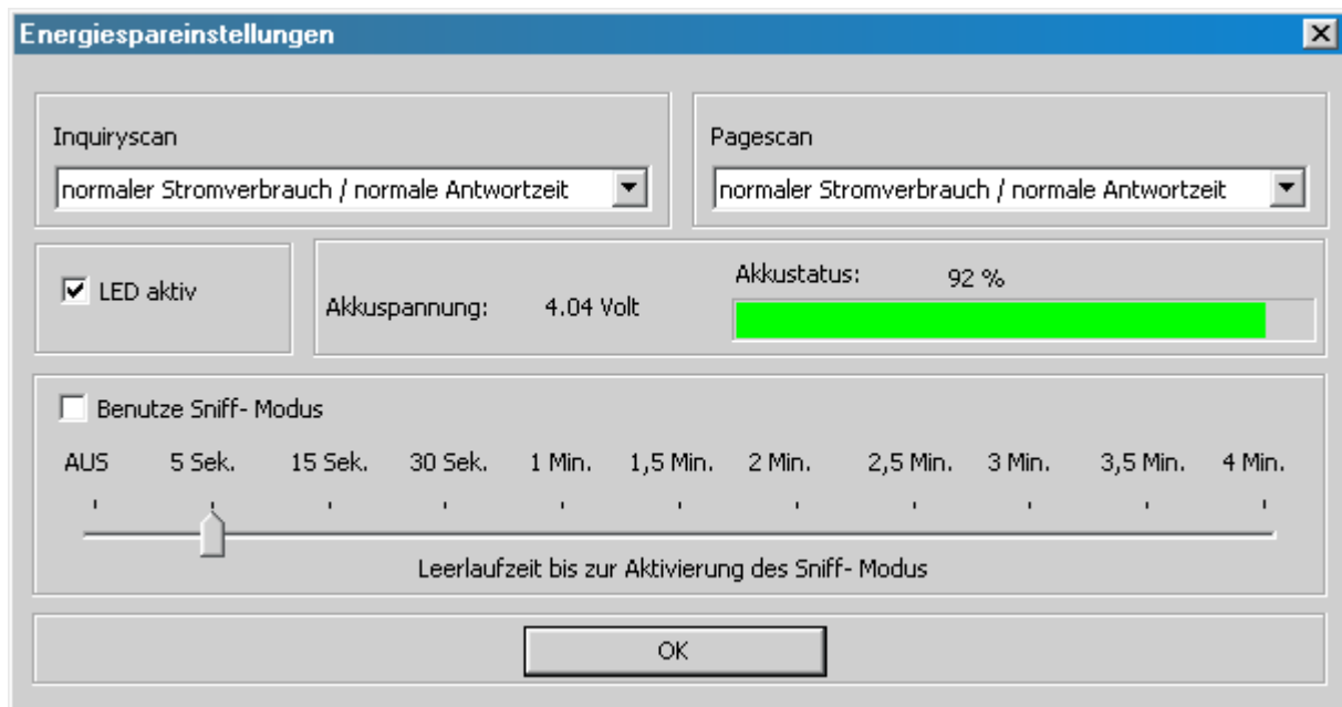
Abbildung 6 Dialog: Energiespareinstellungen
